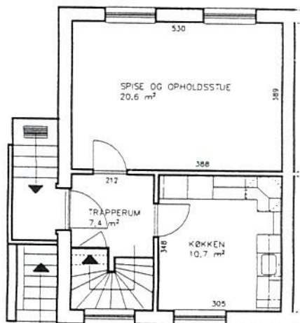
STUEPLAN
