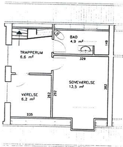
LOFTSPLAN
