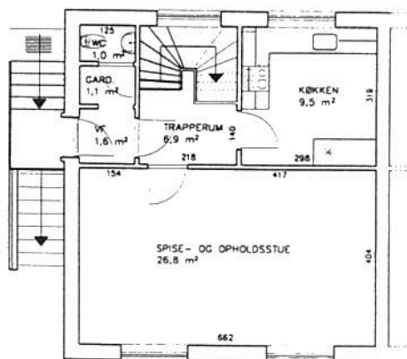
STUEPLAN
