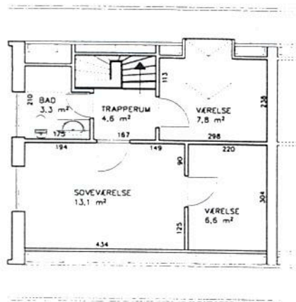
LOFTSPLAN
