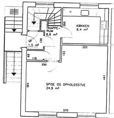
STUEPLAN
