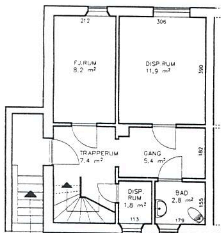
KÆLDERPLAN
