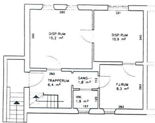
KÆLDERPLAN
